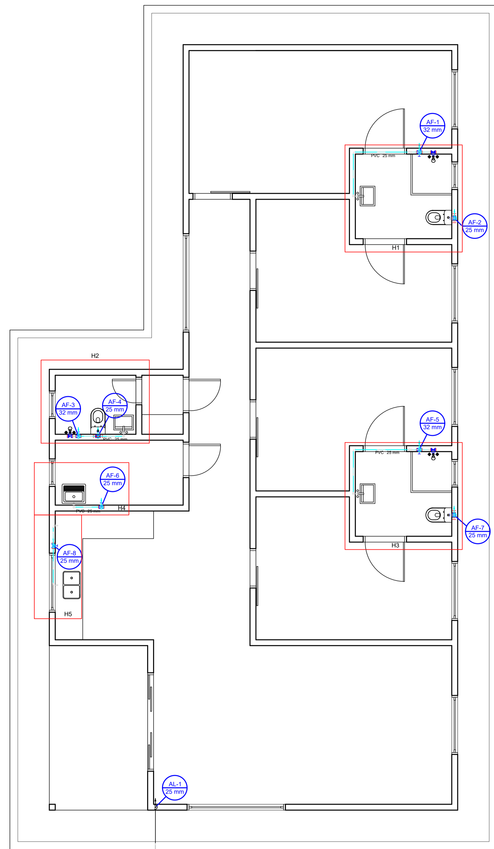
REDE HIDRÁULICA PAV. TÉRREO - CASA 09
