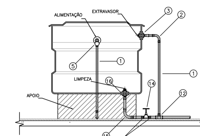
CORTE TRANSVERSAL
