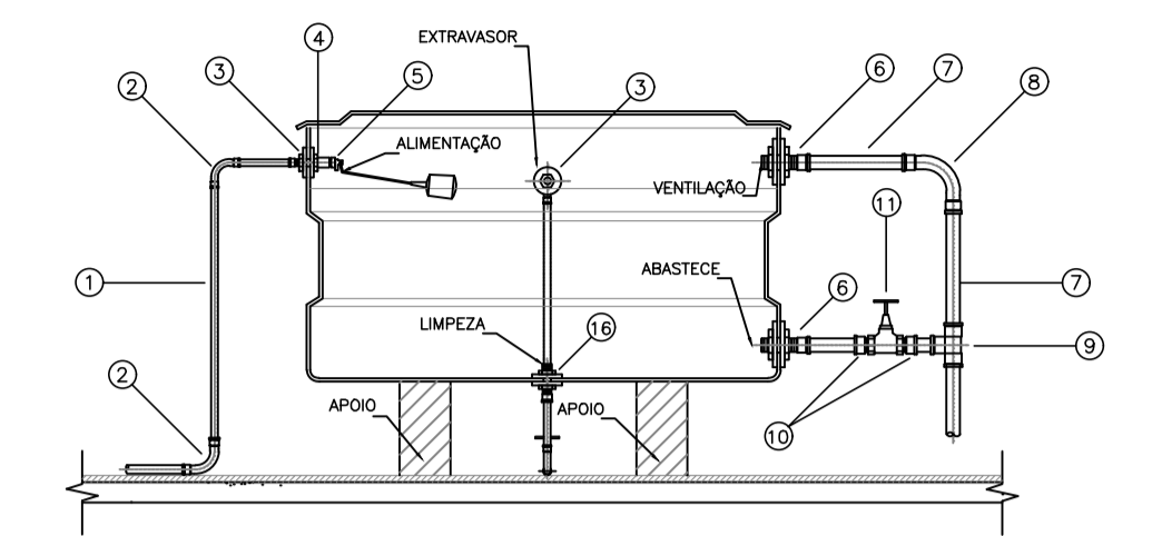
CORTE LONGITUDINAL
