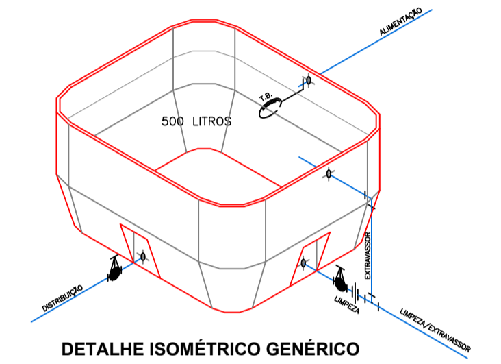
DETALHE ISOMÉTRICO GENÉRICO
